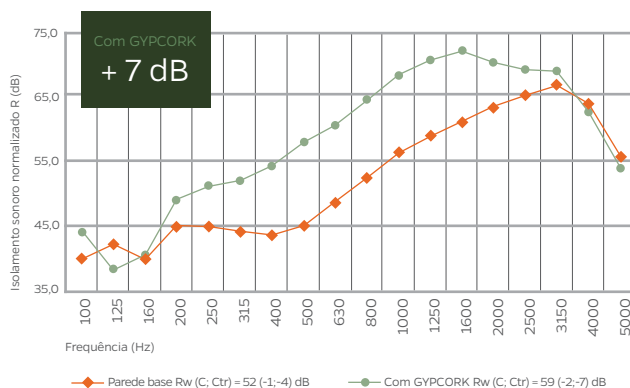
Ensaios ITeCons - Determinação laboratorial do índice de isolamento sonoro para sons de condução aérea, R_w , (normas NP EN 20140-3 e ISO 717-1). ICB 40mm.
