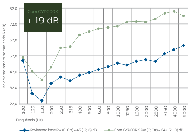
Ensaios ITeCons - Determinação laboratorial do índice de isolamento sonoro para sons de condução aérea, R_w , (normas NP EN 20140-3 e ISO 717-1). ICB 40mm.
