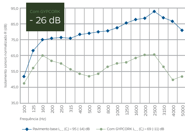
Ensaios ITeCons - Determinação laboratorial do índice de isolamento sonoro para sons de condução por percussão, L_{n,w} , (normas ISO 10140-3 e ISO 717-2). ICB 40mm.
